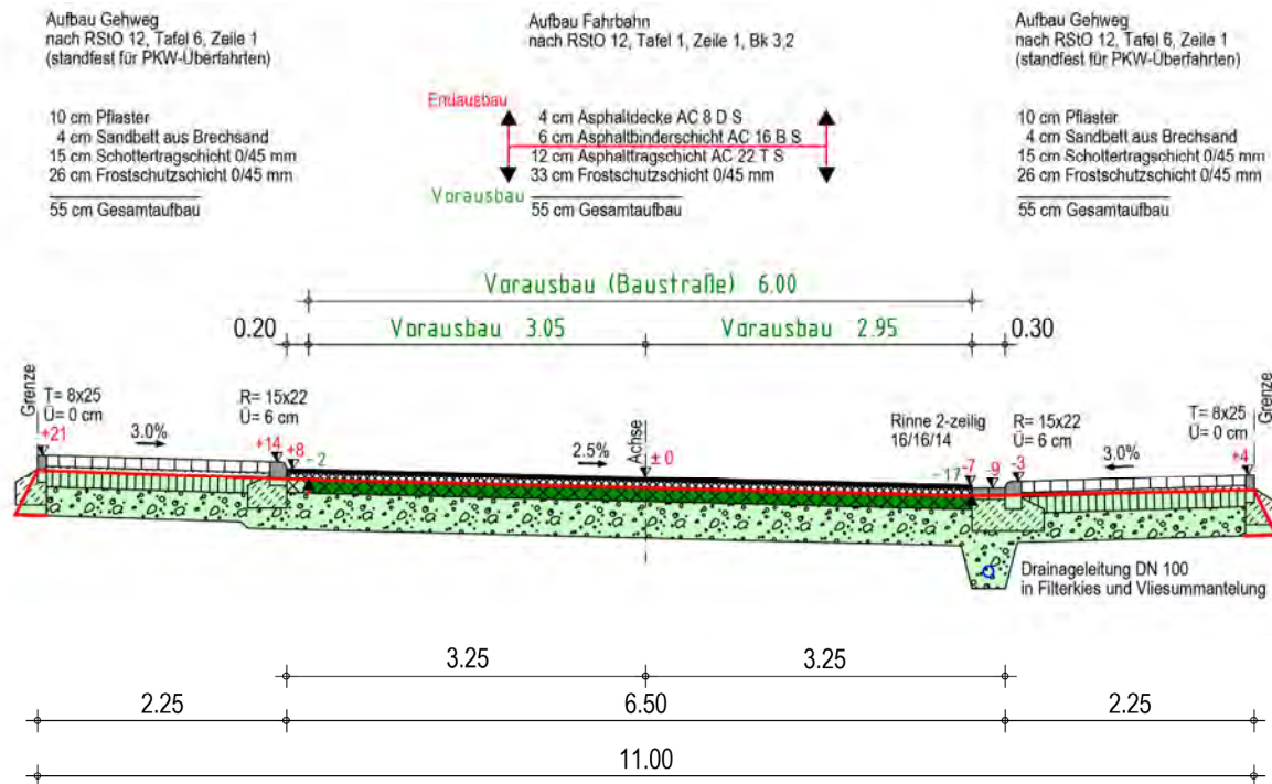
Abbildung 26: Regelquerschnitt Straße 14
